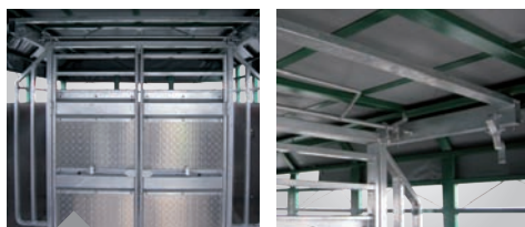
Barrières intérieures 2 battants sur rail avec verrouillage automatique (photo avec option galvanisée)
